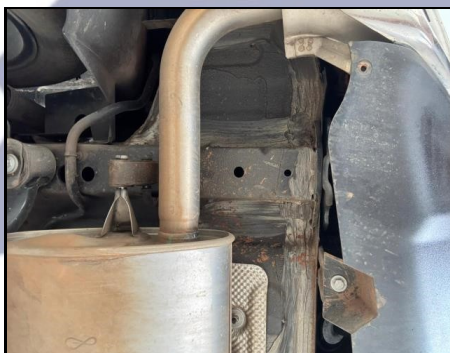
LONGARINA_TRASEIRA_ESQUERDA
